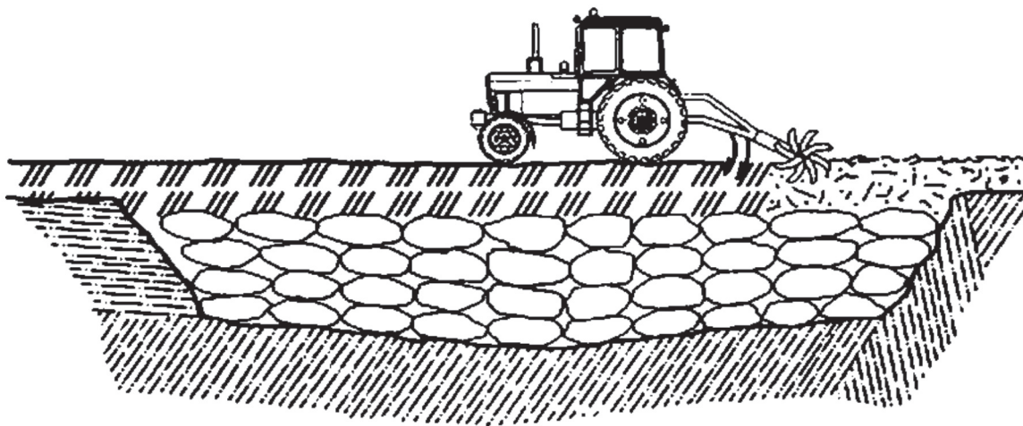
Рисунок А.6 — Операция удаления органических остатков и перемешивания вместе с модификатором свойств грунтов и минеральным вяжущим верхнего слоя грунта обваловки сооружения, предназначенного для срочного захоронения трупов
