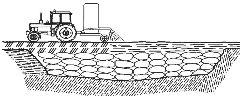
Рисунок А.8 — Операция увлажнения верхнего слоя грунта обваловки сооружения, предназначенного для срочного захоронения трупов, усиленного модификатором свойств грунтов и минеральным вяжущим с помощью поливальной машины
