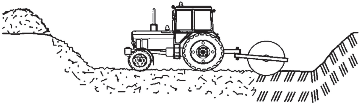
Рисунок А.3 – Операция уплотнения донного слоя грунта котлована сооружения, предназначенного для срочного захоронения трупов, усиленного модификатором свойств грунтов и минеральным вяжущим с помощью катка
