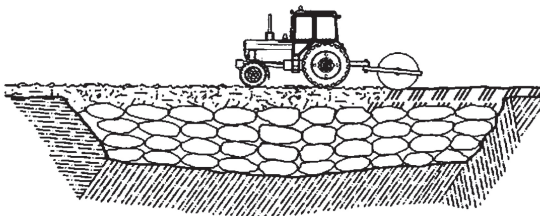
Рисунок А.6 — Операция удаления органических остатков и перемешивания вместе с модификатором свойств грунтов и минеральным вяжущим верхнего слоя грунта обваловки сооружения, предназначенного для срочного захоронения трупов
